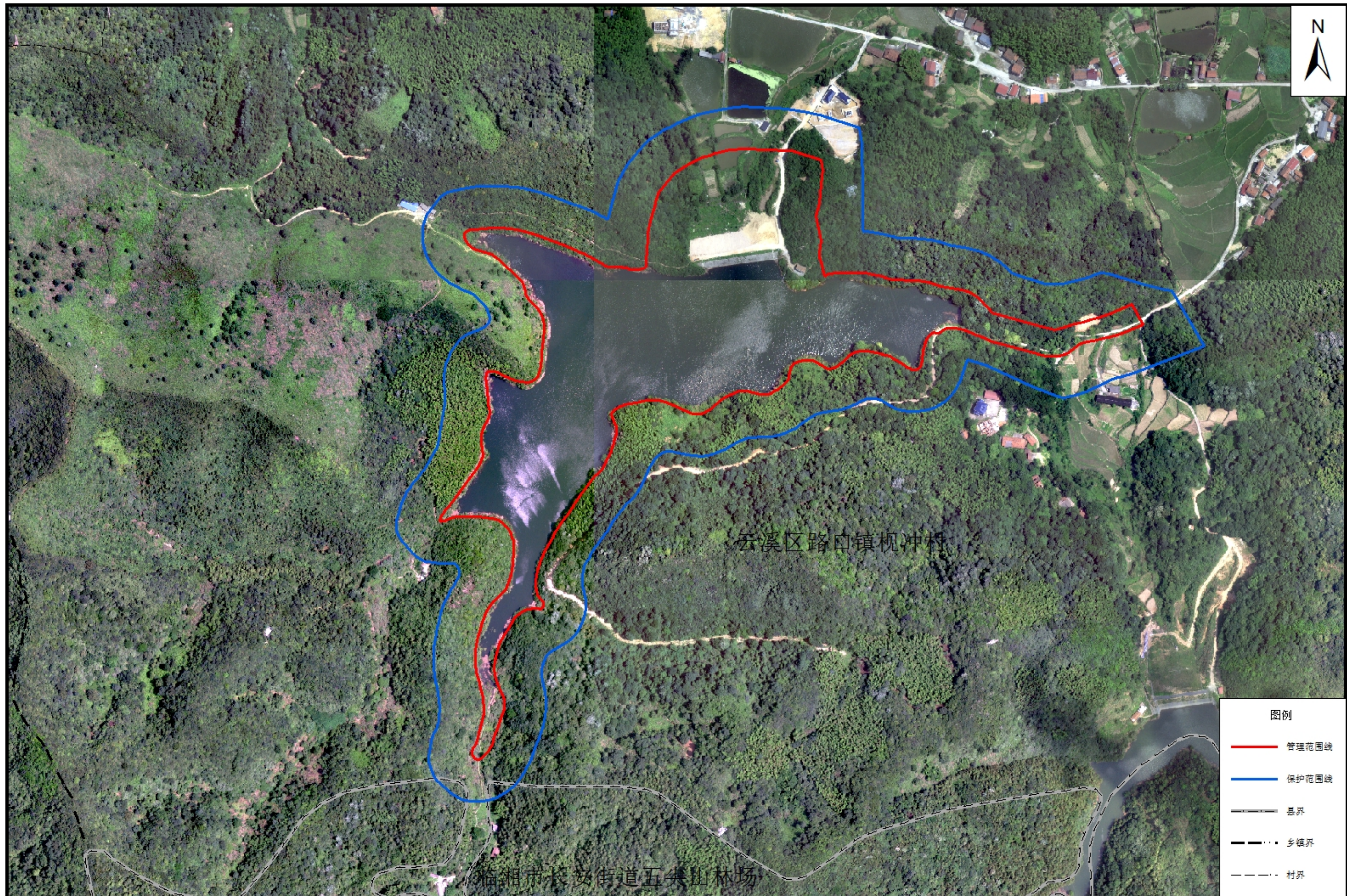
柃冲水库管理与保护范围划界成果示意图
