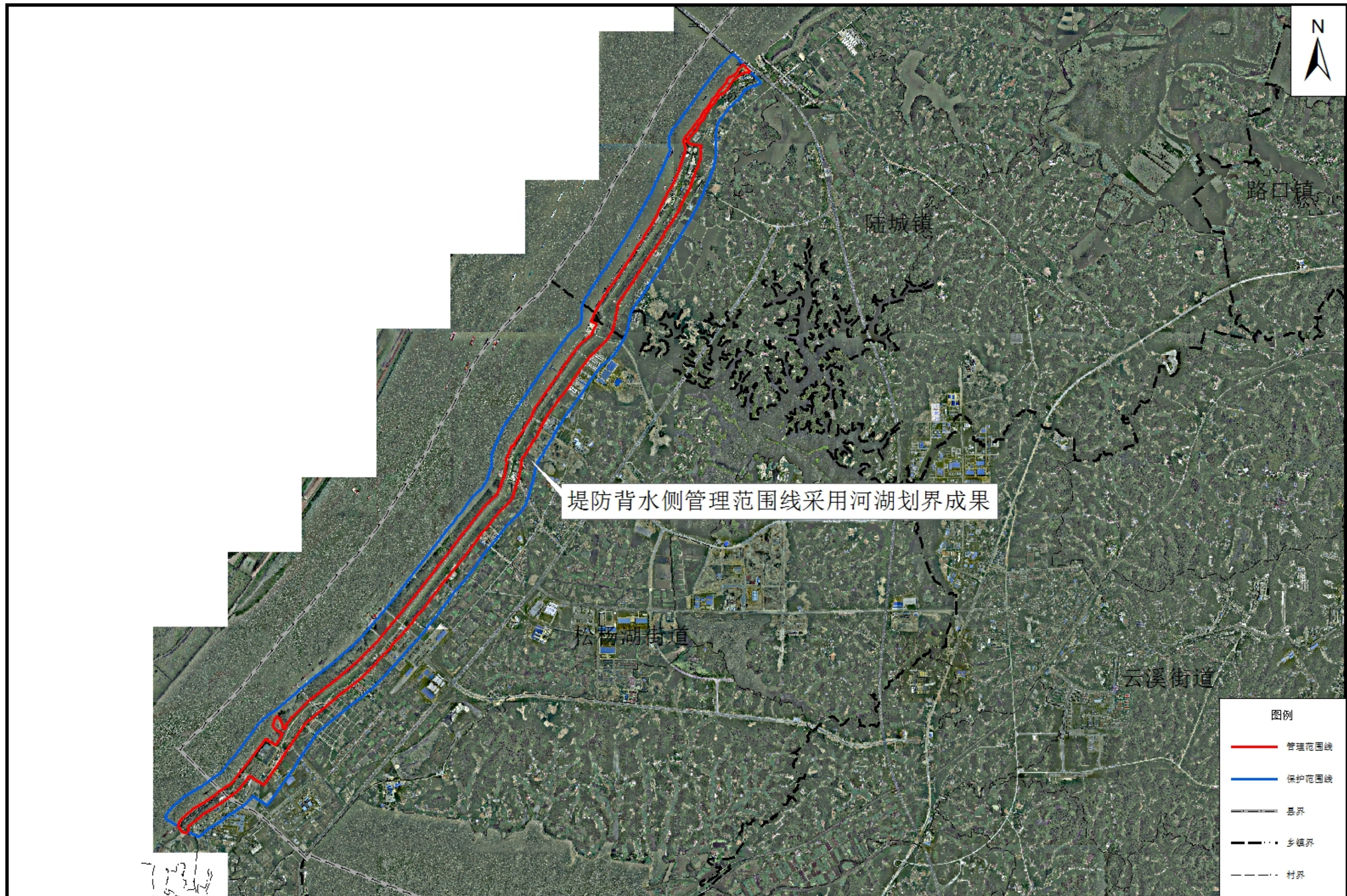
长江干堤——云溪区永济垸段管理与保护范围划界成果示意图
