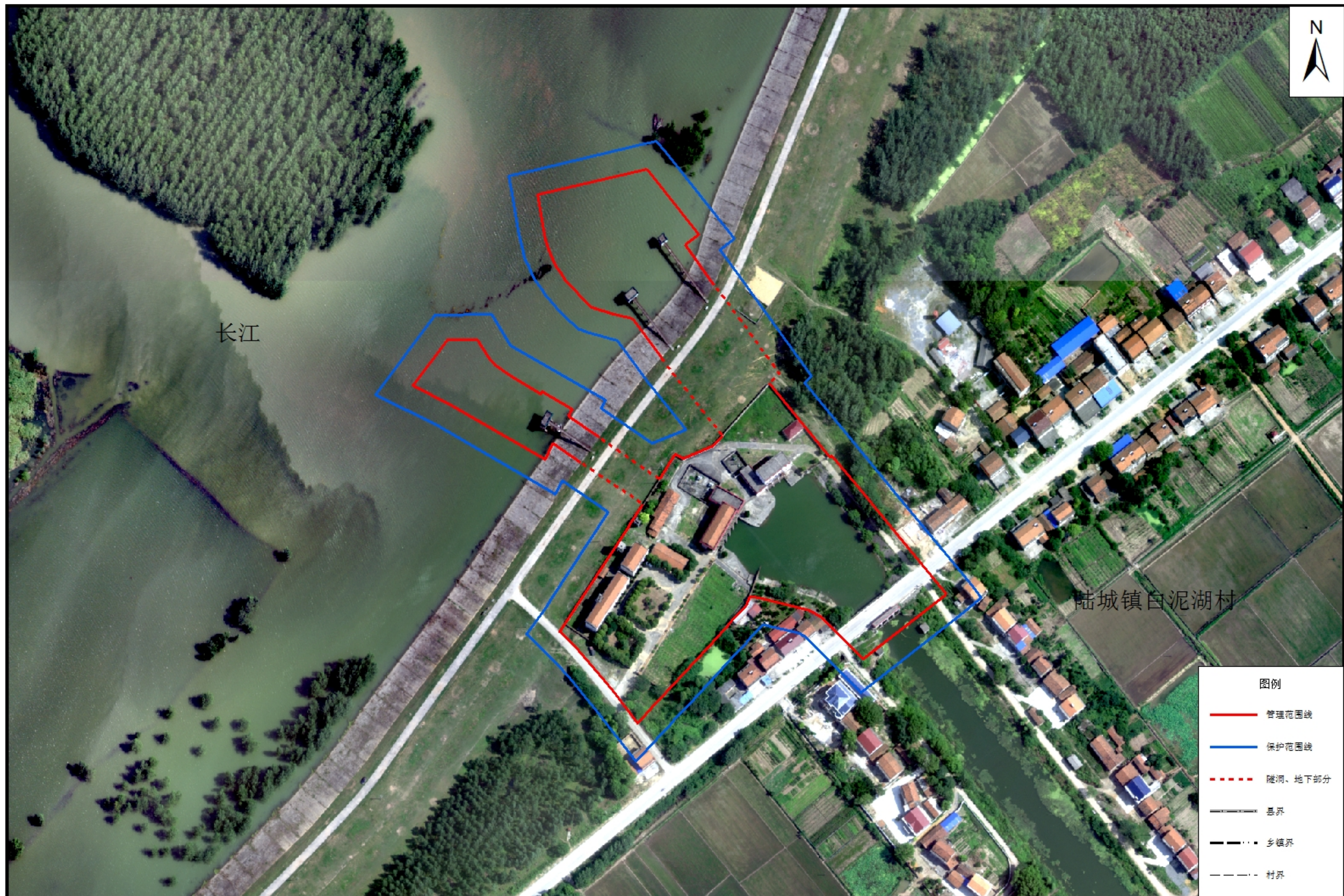
新设电排、土矾头电排管理与保护范围划界成果示意图
