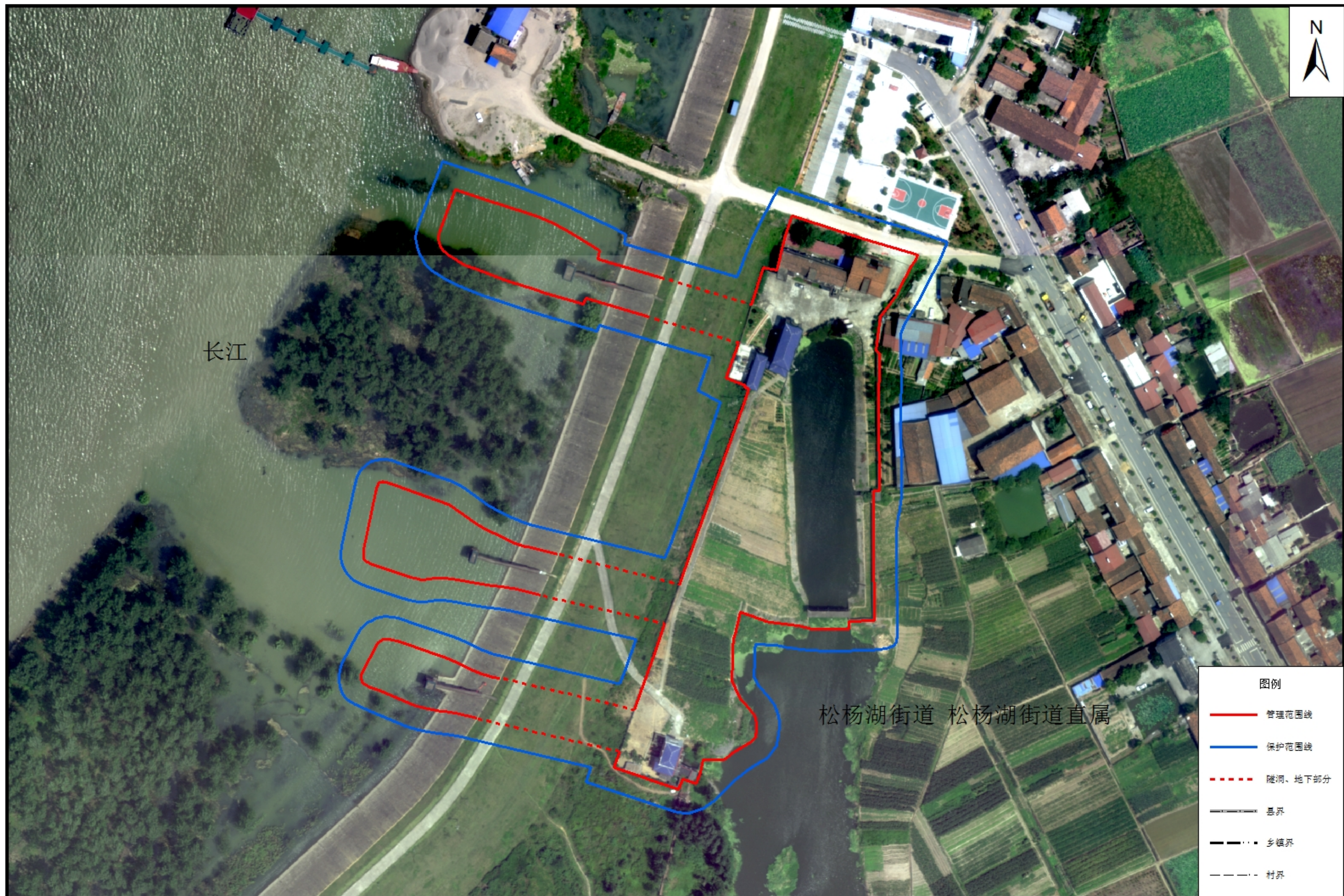
象骨港电排管理与保护范围划界成果示意图
