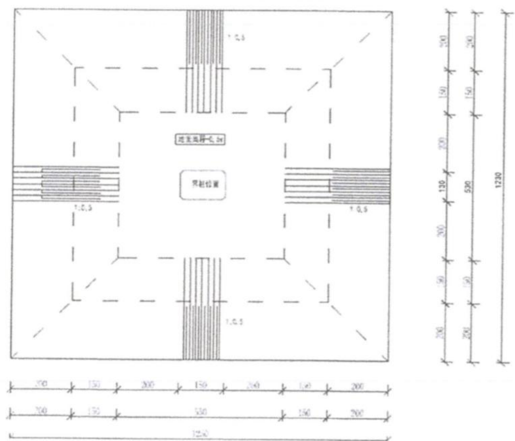
图 6-2 界桩平面图
