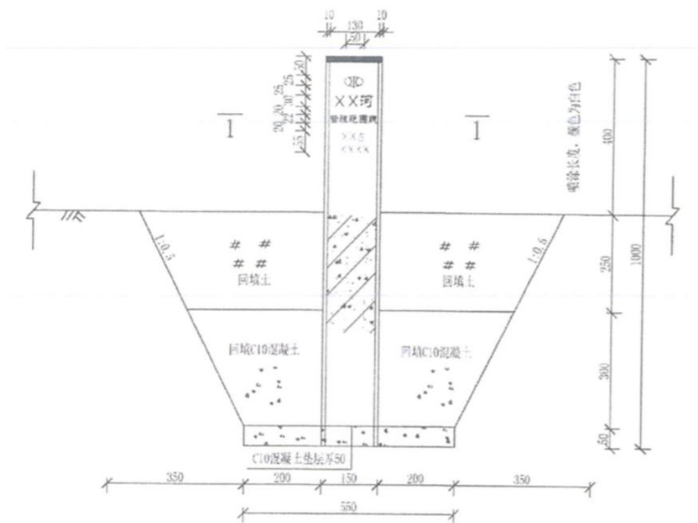
图 6-1 界桩结构图
