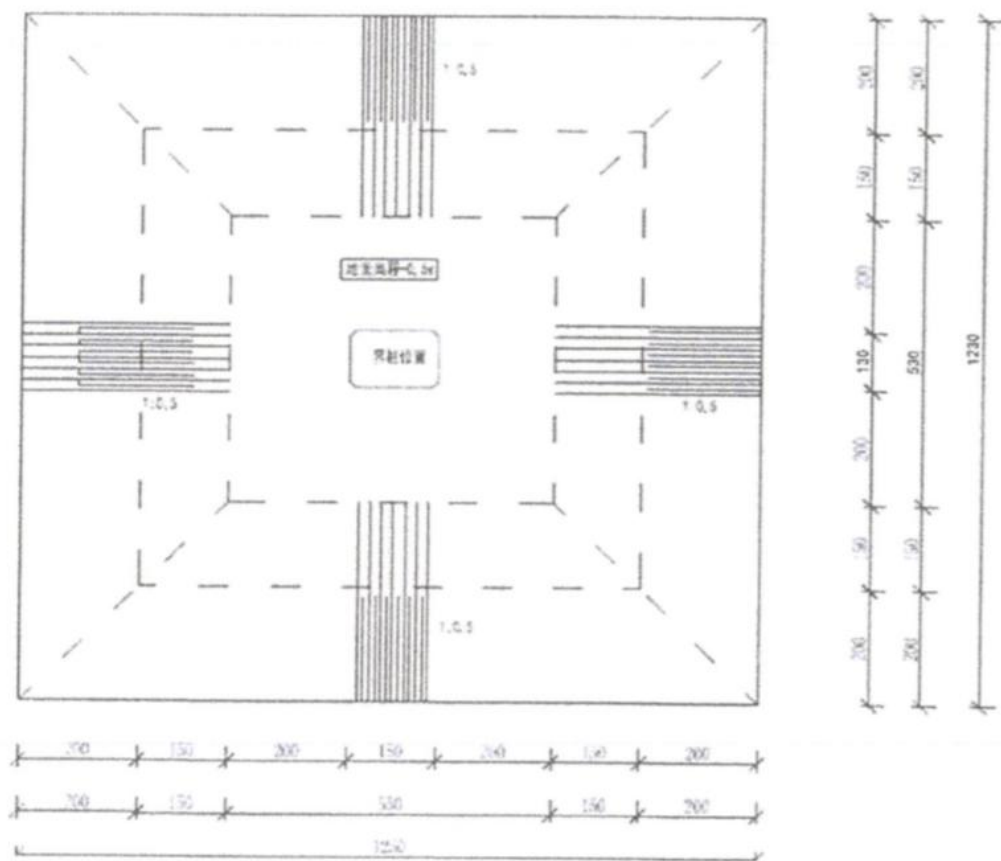
图 6-2 界桩平面图
