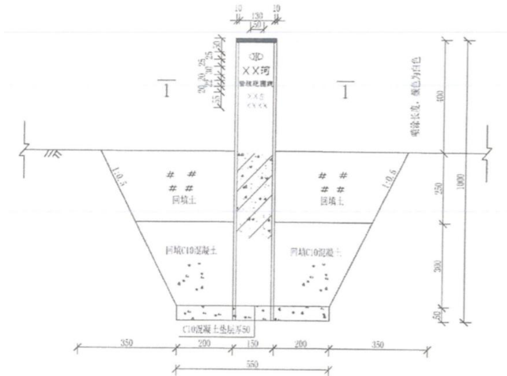
图 6-1 界桩结构图
