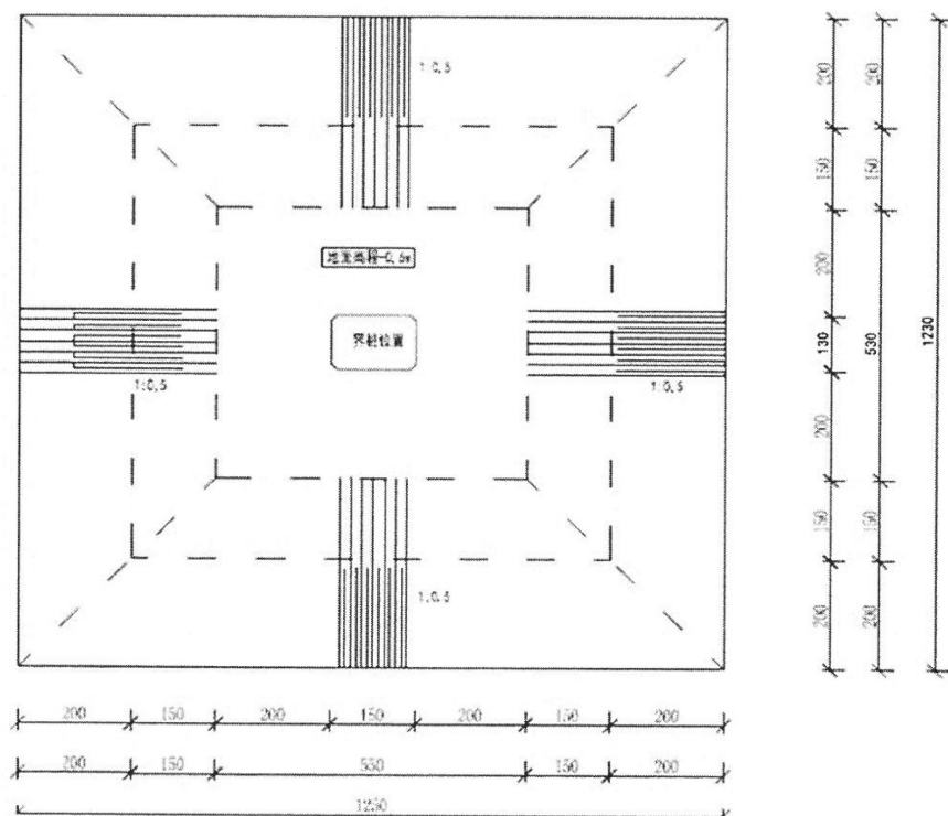
图 6.2-2 管理范围界桩平面图
