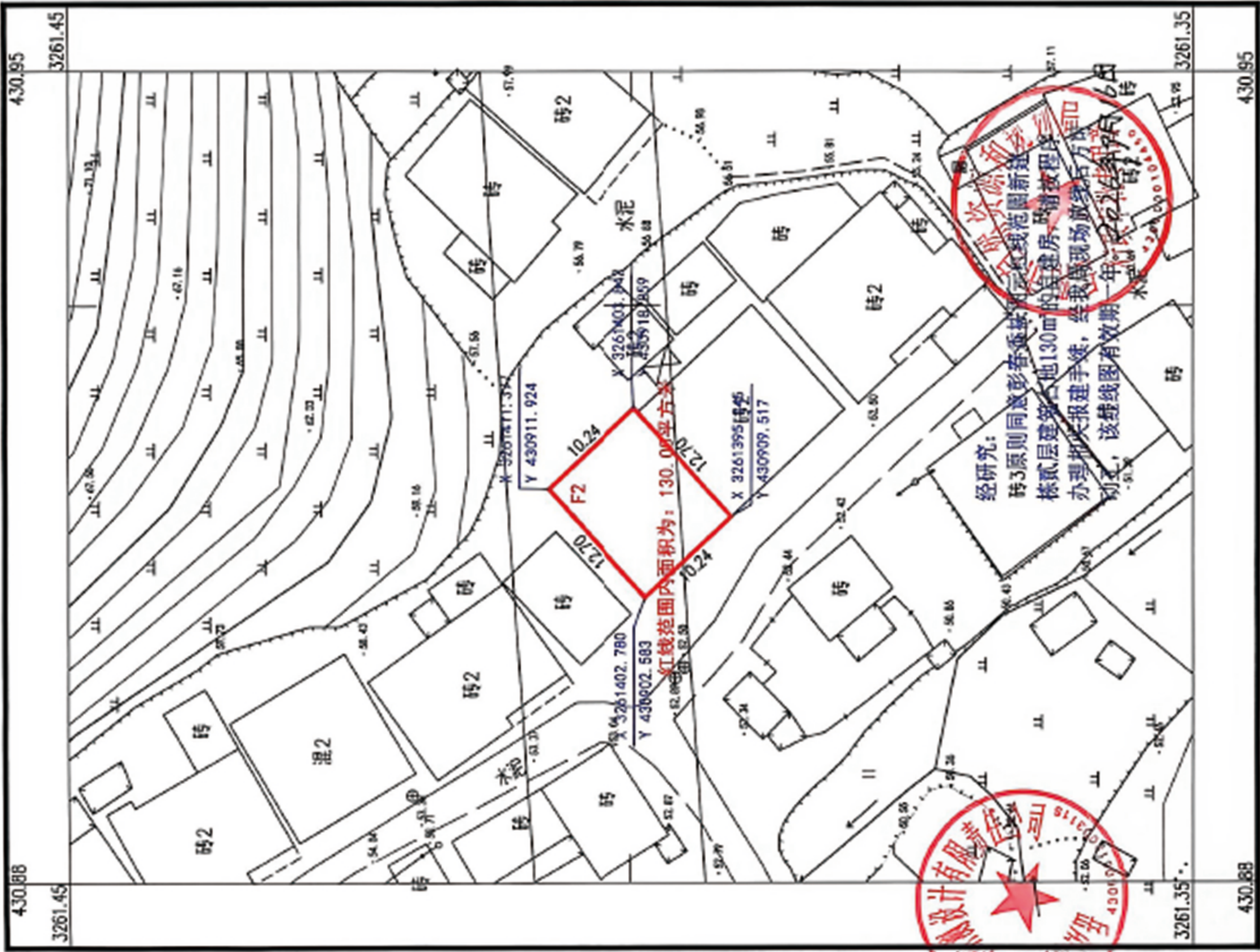
彭春香房屋红线图
